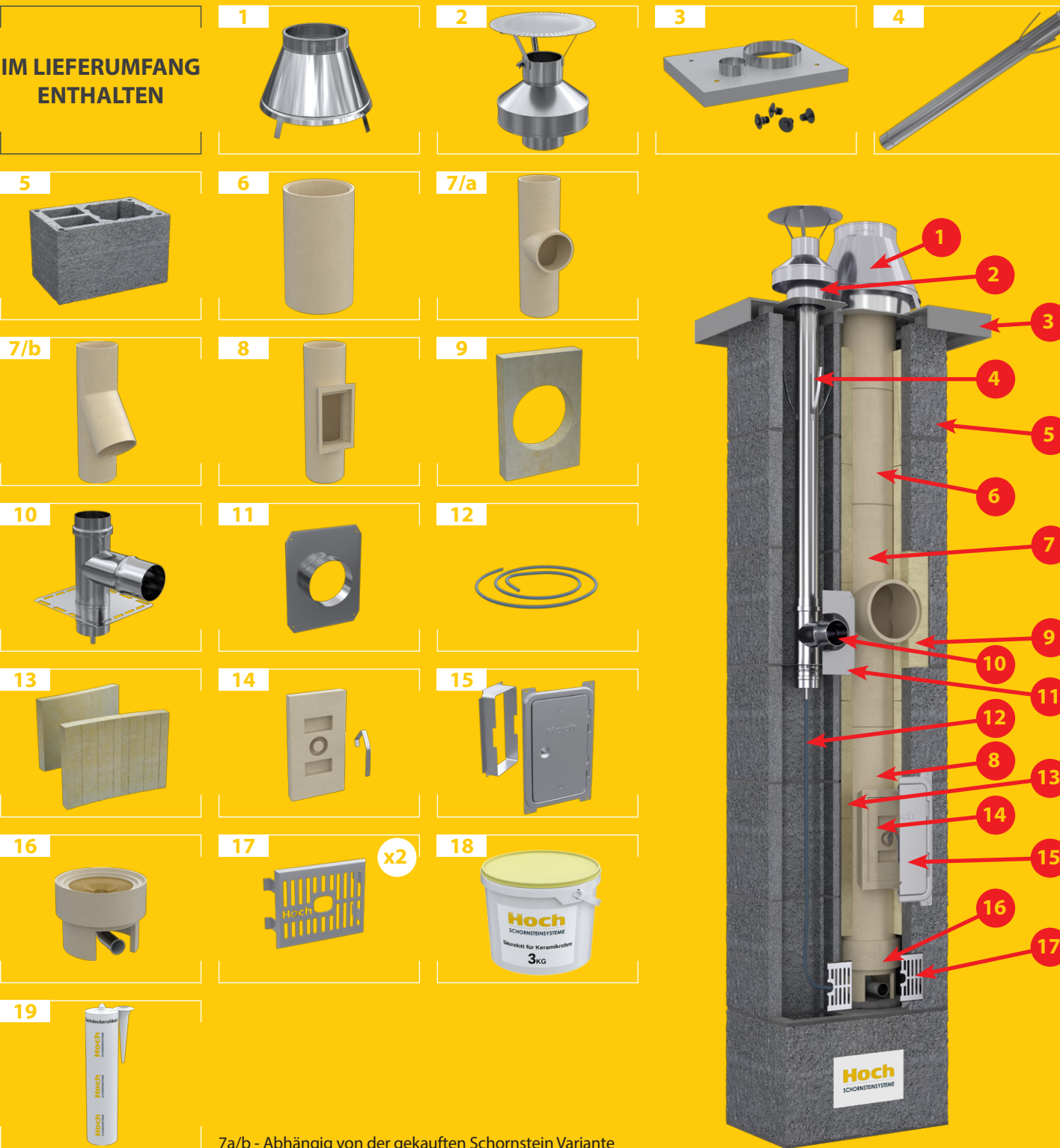
7a/b - Abhängig von der gekauften Schornstein Variante
